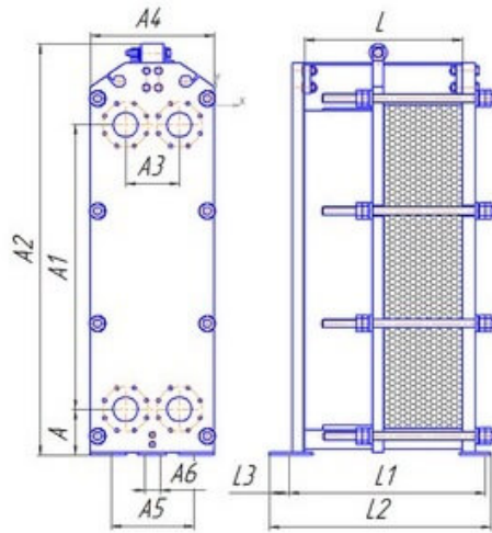
Теплообменник Этра ЭТ-070
